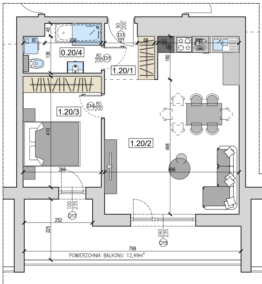
PIĘTRO I SCHEMAT KONDYGNACJI
