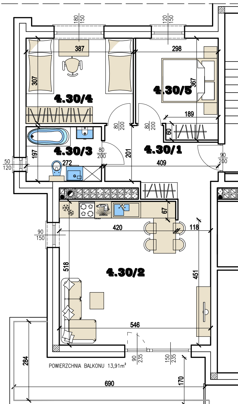
PIĘTRO 4 SCHEMAT KONDYGNACJI
