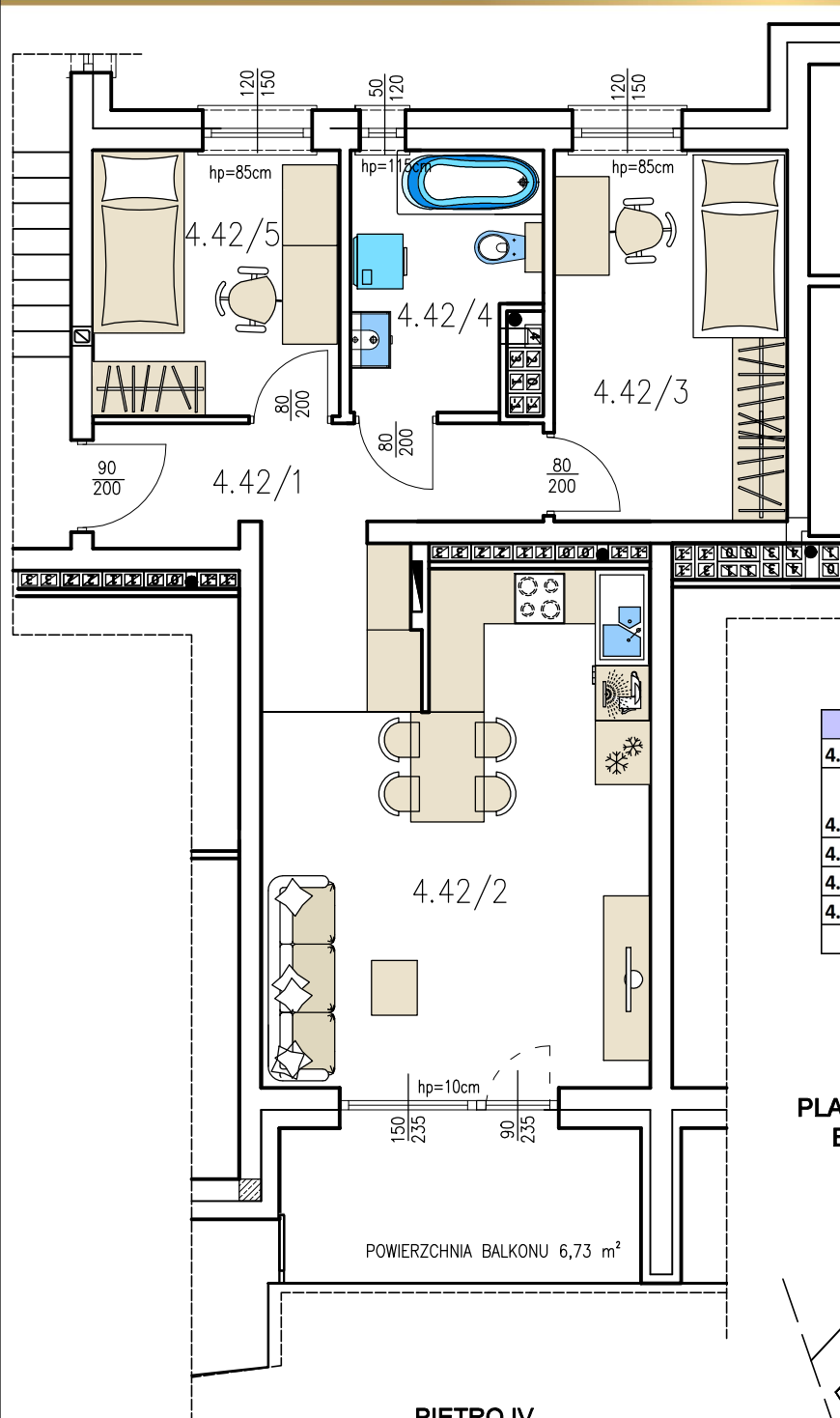
PIĘTRO IV SCHEMAT KONDYGNACJI
