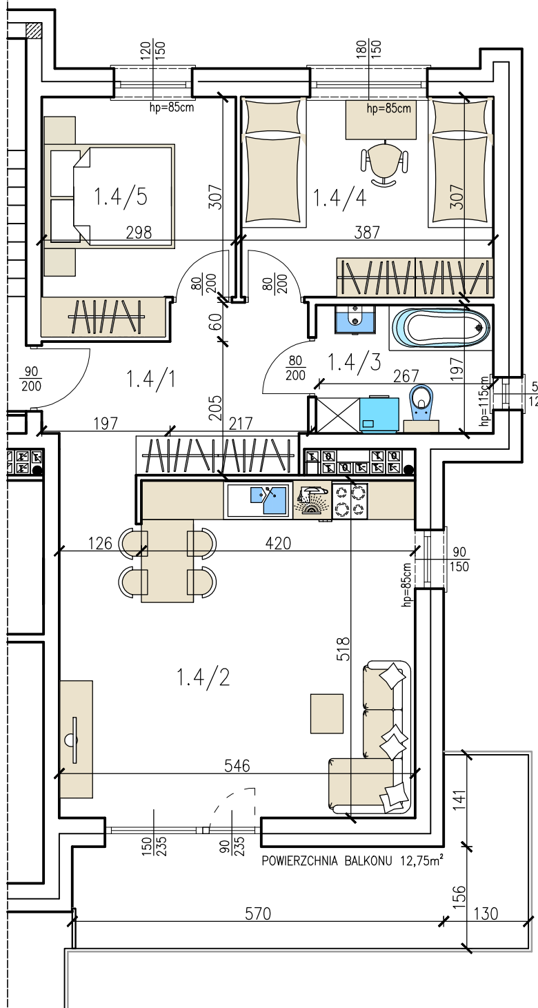
I PIĘTRO SCHEMAT KONDYGNACJI
