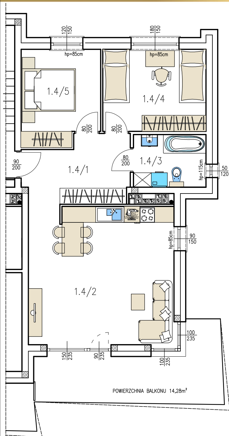
PIĘTRO I SCHEMAT KONDYGNACJI
