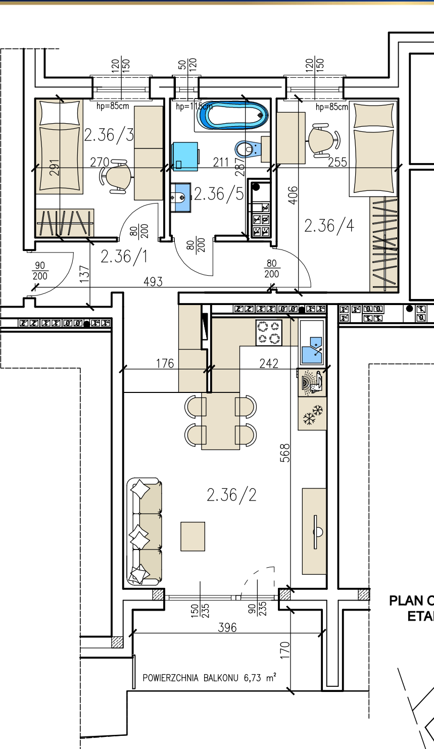
PIĘTRO II SCHEMAT KONDYGNACJI
