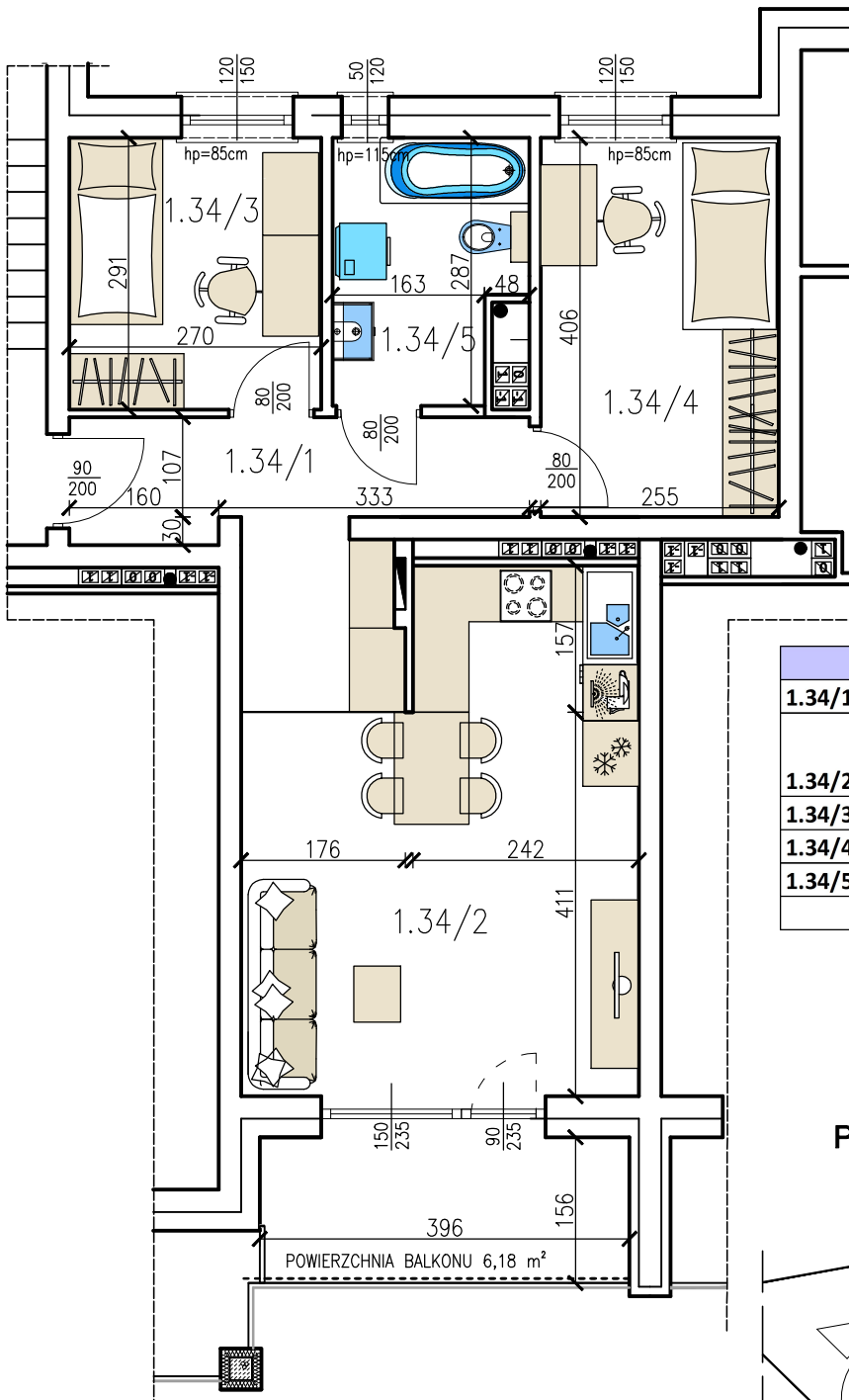
I PIĘTRO SCHEMAT KONDYGNACJI
