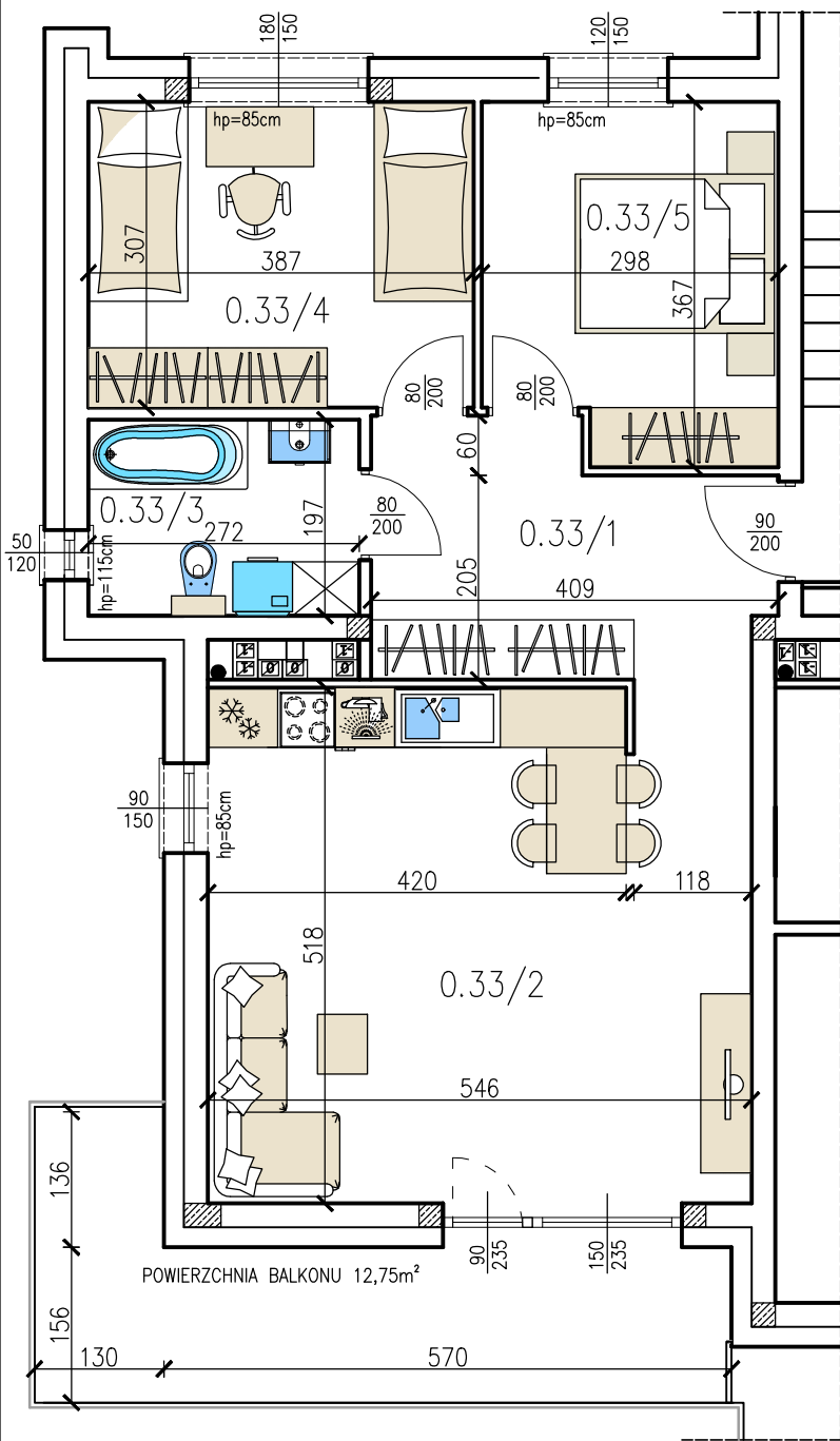
PARTER SCHEMAT KONDYGNACJI
