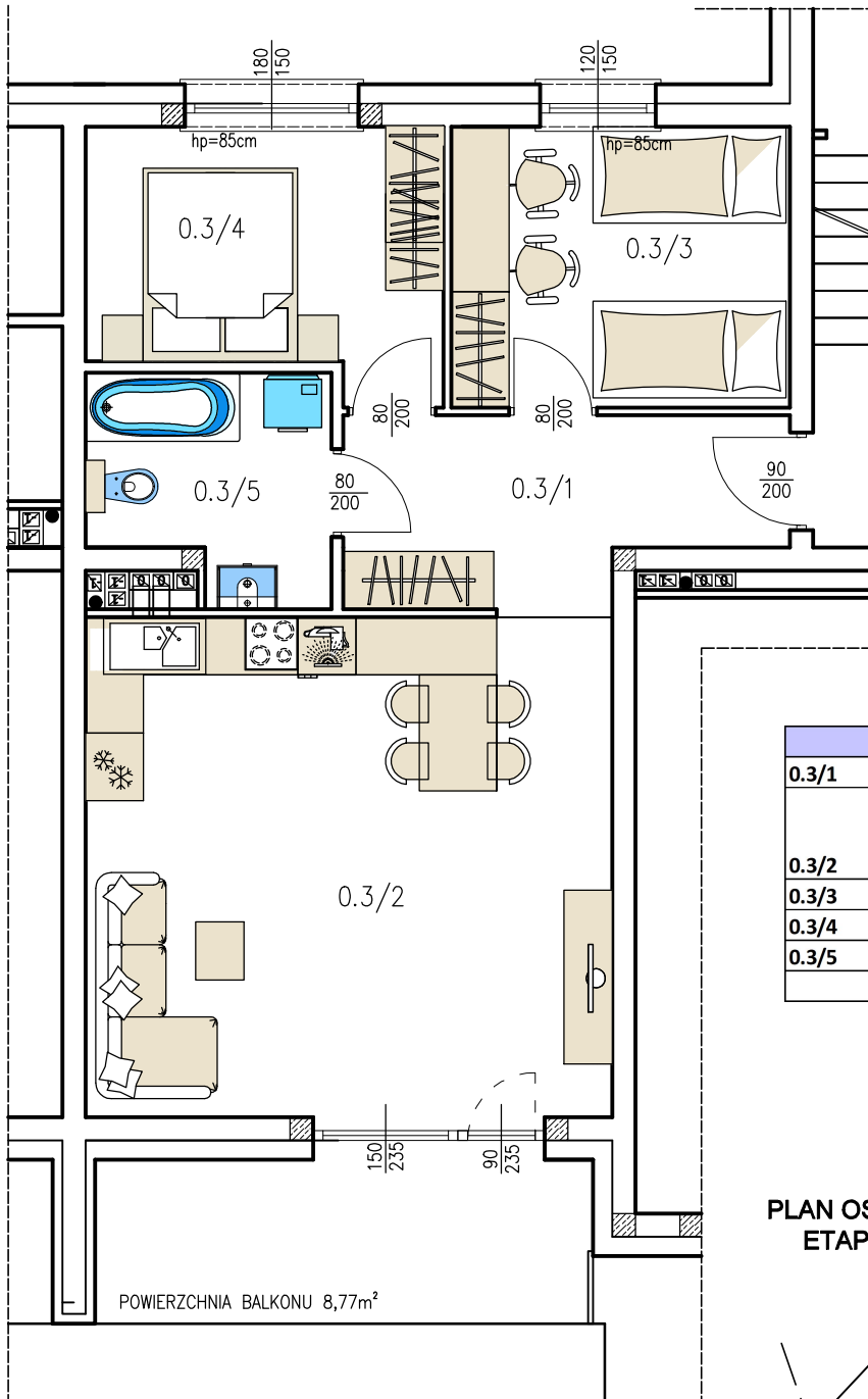
PARTER SCHEMAT KONDYGNACJI
