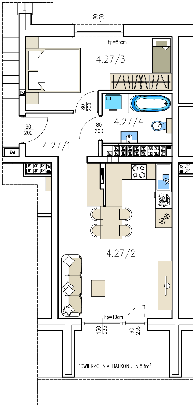
PIĘTRO IV SCHEMAT KONDYGNACJI
