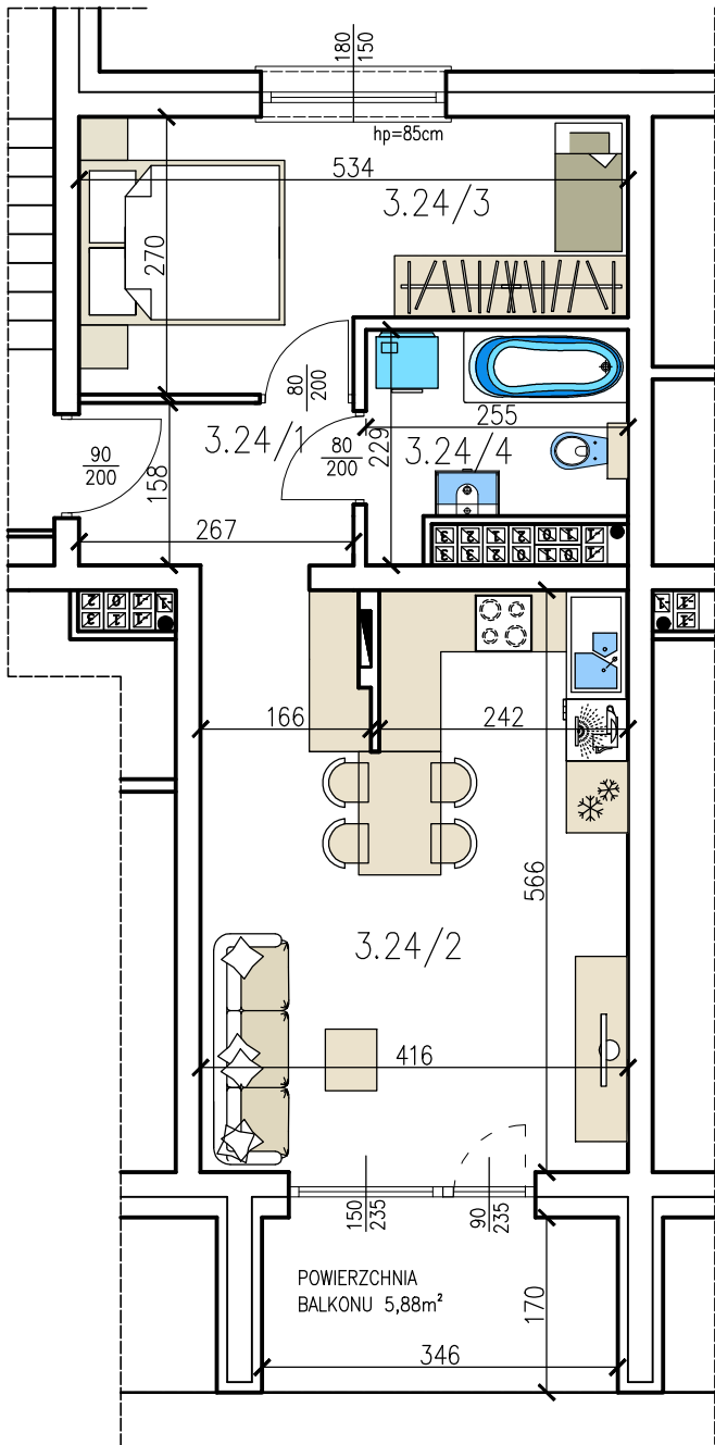
PIĘTRO III SCHEMAT KONDYGNACJI
