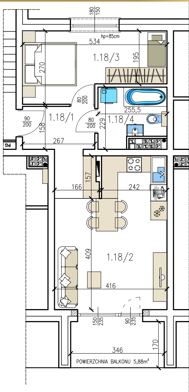
PIĘTRO I SCHEMAT KONDYGNACJI
