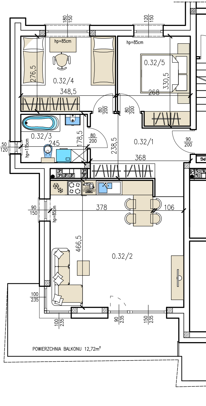
PARTER SCHEMAT KONDYGNACJI
