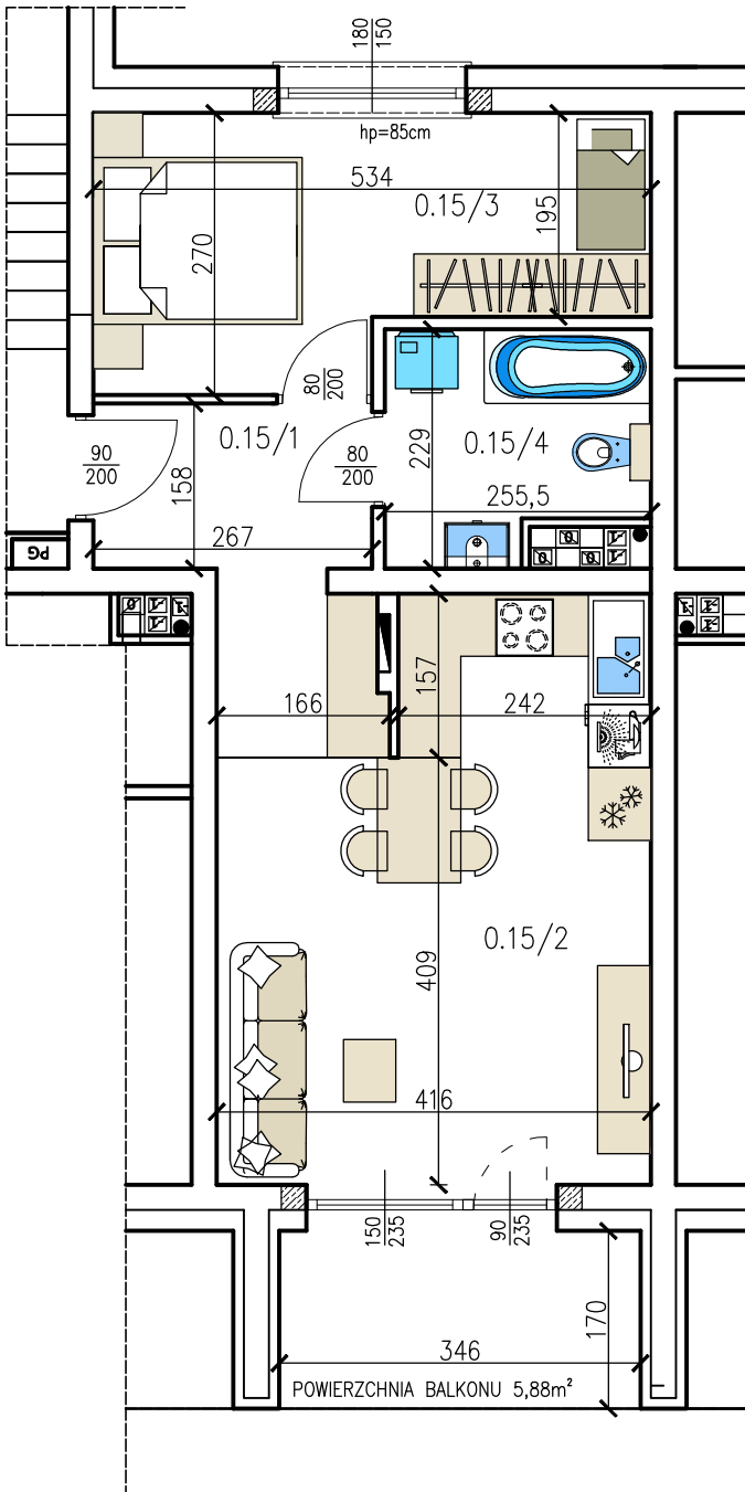
PARTER SCHEMAT KONDYGNACJI
