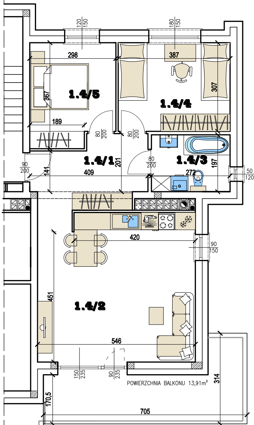
PIĘTRO 1 SCHEMAT KONDYGNACJI
