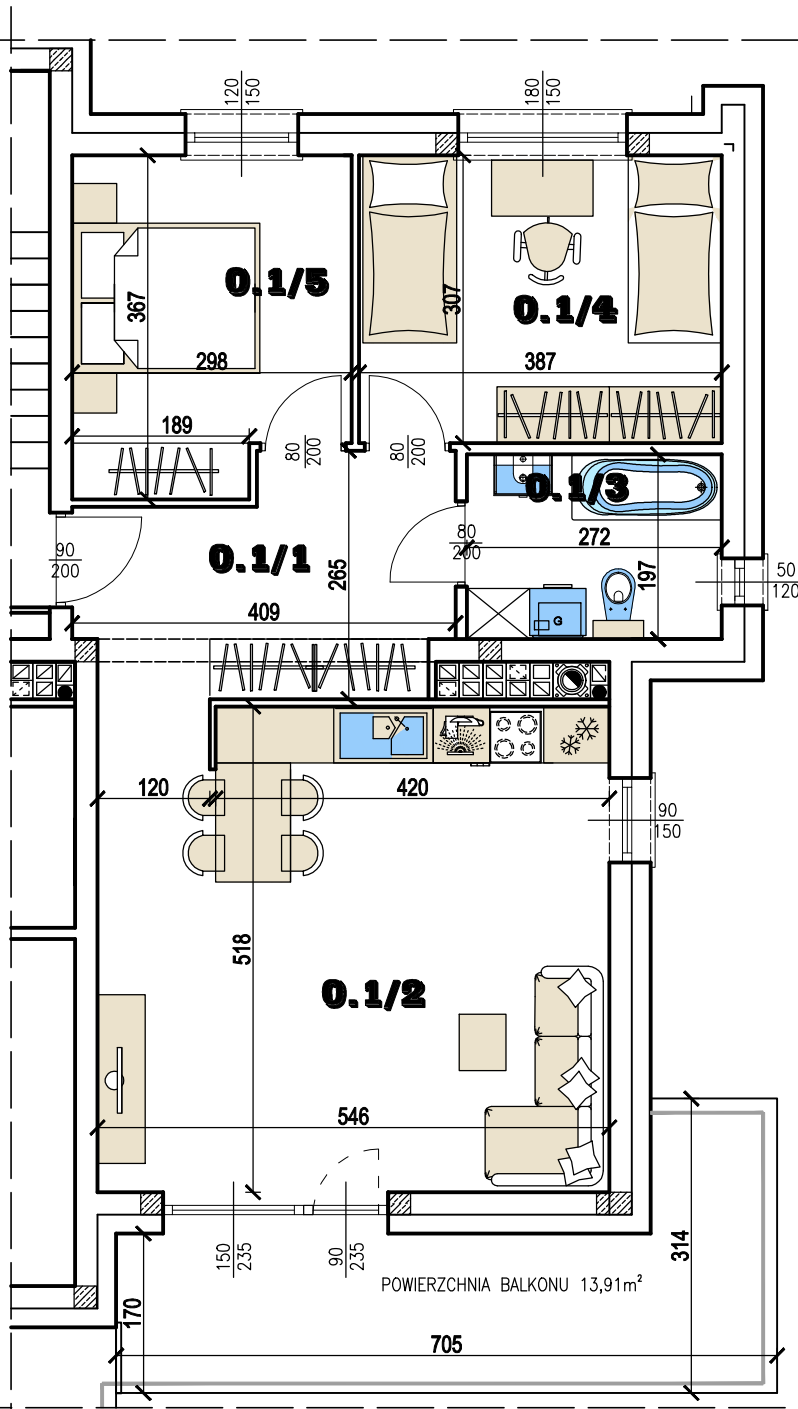
PARTER SCHEMAT KONDYGNACJI
