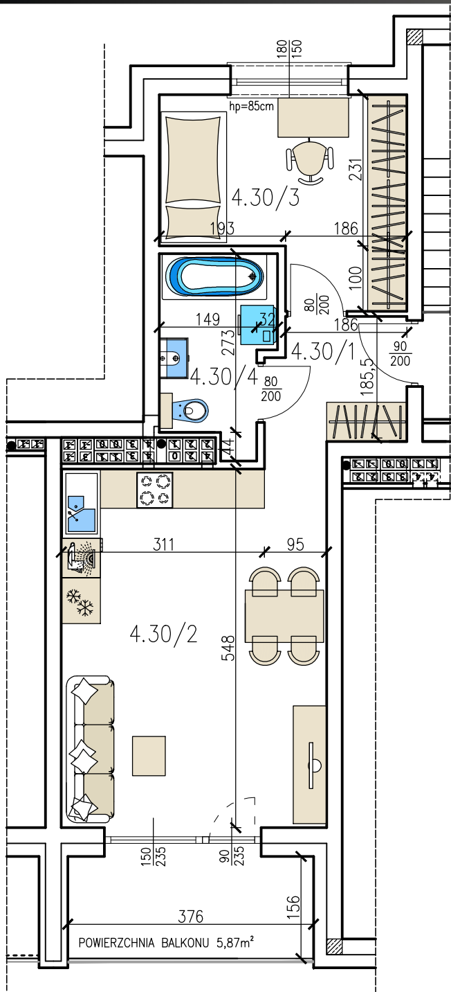
IV PIĘTRO SCHEMAT KONDYGNACJI
