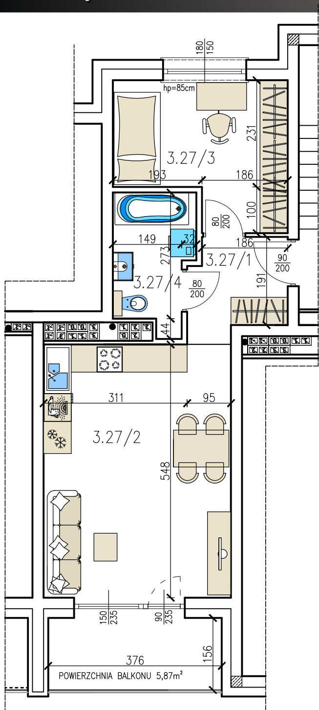
III PIĘTRO SCHEMAT KONDYGNACJI
