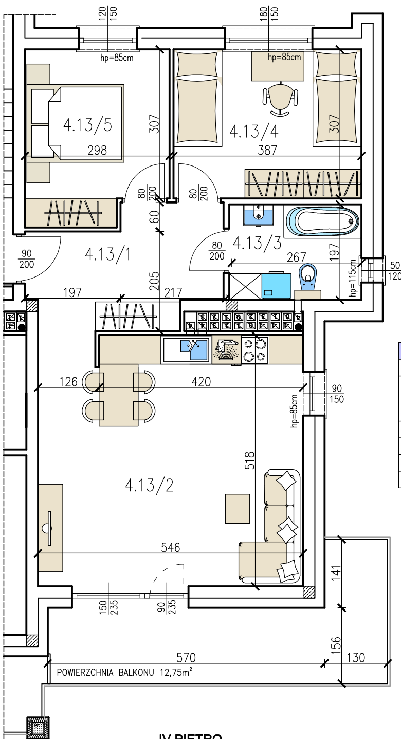
IV PIĘTRO SCHEMAT KONDYGNACJI
